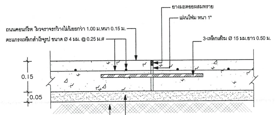
รูปตัดถนน C
